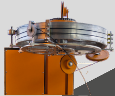
Düzgün kangal ünitesi Coiling pallet Paleta enrollable منصة التبريد
